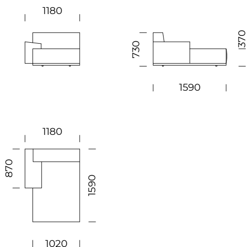
Szezlony lewy 1 / Left chaise longue 1
