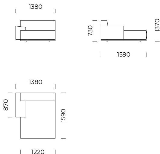
Szezlony lewy 2 / Left chaise longue 2
