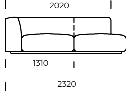
Chaise longue right
