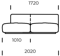
Backres sofa module left
