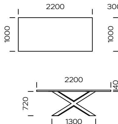
Tisch Cruzar 2200 x 1000
