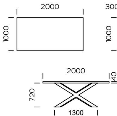
Tisch Cruzar 2000 x 1000
