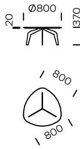
Triangular table FEZA 800
