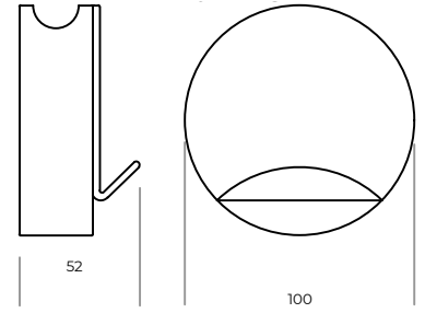
Wieszak drewniany Ø100
